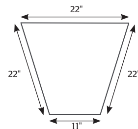
11 Wedge Table 22"w X 22"d X 25"h
